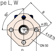
Flanschzähler
