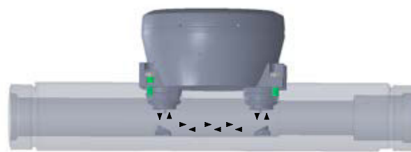
Das Ultraschallprinzip
