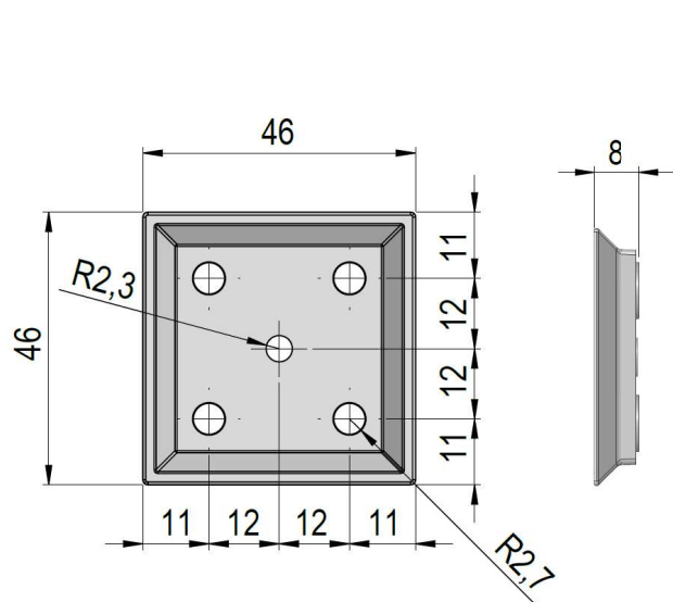
Abb. 10: Wandhalterung
